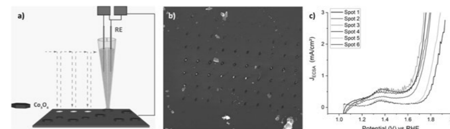
(5) a) Schematische Darstellung der sequentiellen Scanning Electrochemical Cell Microscopy (SECCM)-Untersuchung einer mit Co 3 O 4 -Partikeln modifizierten Glaskohlenstoffplatte. b) Rasterelektronenmikroskop (SEM)-Abbildung des SECCM-Scans. c) Voltammetrische Scans an unterschiedlichen Tropfenlandungsstellen für die Untersuchung der Sauerstoffevolutionsaktivität.
