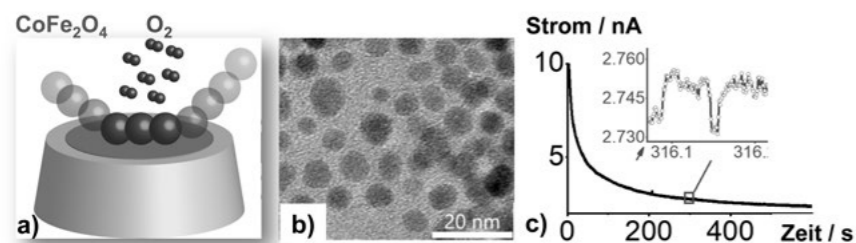
(4) a) Schematische Darstellung der Sauerstoffentwicklung an einem einzelnen CoFe 2 O 4 -Nanopartikel während elektrochemischer Einschlagsexperimente (nano-impact electrochemistry) an einer Mikroelektrode. b) TEM-Abbildung der untersuchten Nanopartikel. c) Der Strom-Zeit Verlauf der Elektrode zeigt die katalytische Aktivität nacheinander auftretender Partikel in Form charakteristischer Stromstufen.
