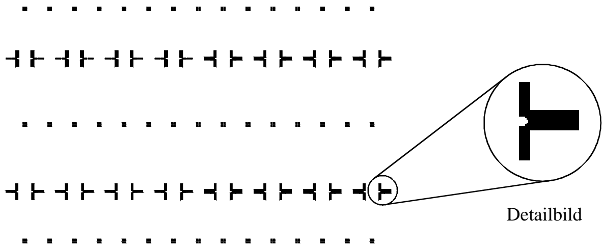
Maske metall1-Ohm
