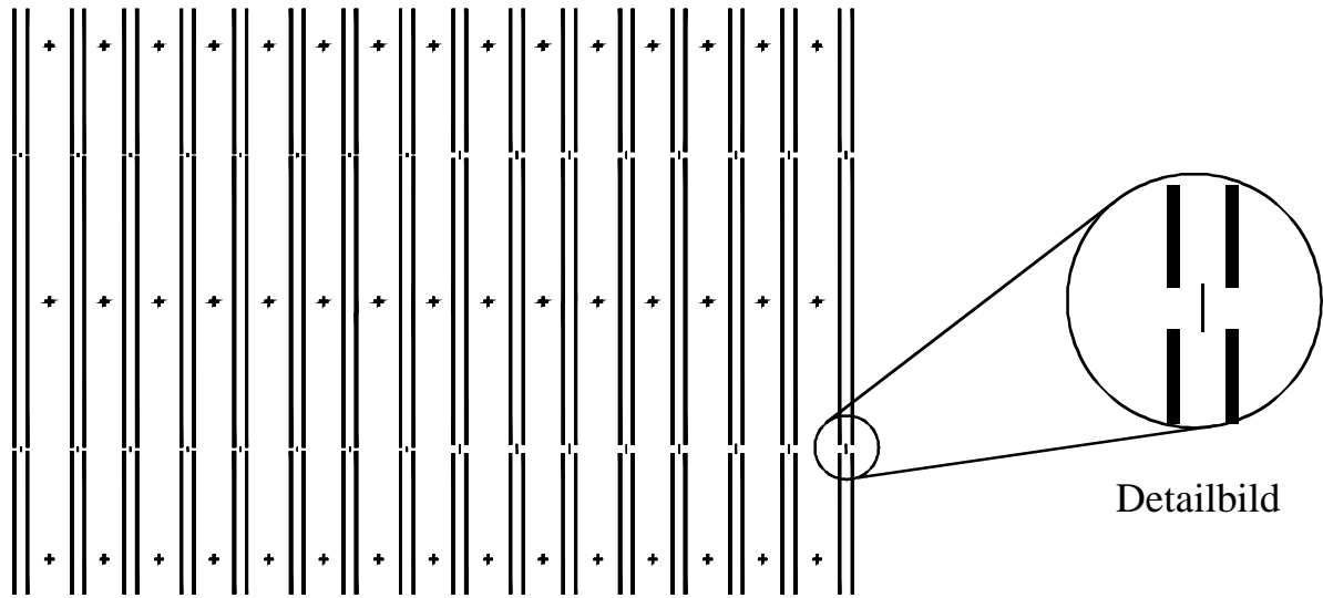
Maske aetz-1-pos
