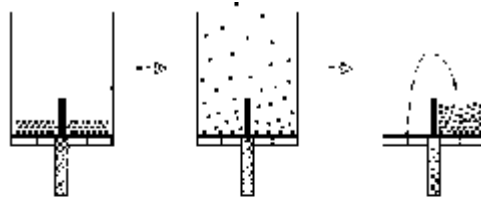
Abb. 13: Die flache Verteilung ist instabil und führt zu einer Anreicherung der Glaskugeln in einer der beiden Zellen.
