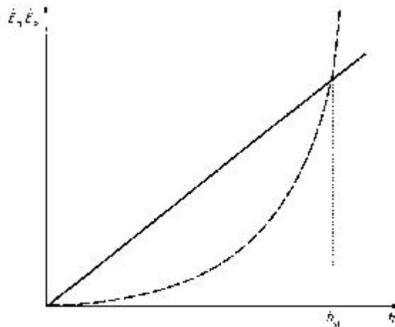
Abb. 15. Verhalten der Energieströme E_D und E_P als Funktion der Höhe eines gegebenen Haufens.
