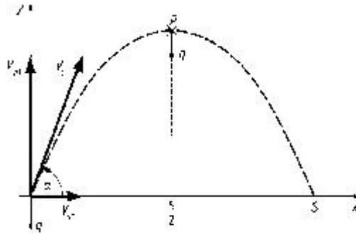
Abb. 16. Schiefer Wurf: Flugparabel und Komponentenzerlegung der Anfangsgeschwindigkeit.
